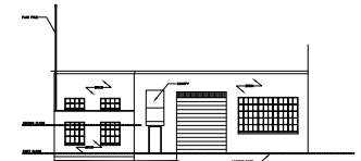
5 EXISTING ELEVATION
